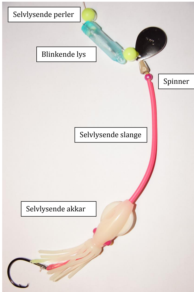
Figur 1. Sluk brukt av fritidsfiskere i norske farvann for bunnfisk som torsk, hyse, brosme, lange og lysing. I tillegg til en krok for å feste naturlig eller kunstig agn (eller begge deler), består utstyret av byttedyr-etterlikninger (akkar), visuelle stimuli (rør, perler og blinkende lys) og spinner (bevegelses- og lydstimuli). Ved å feste spinneren i nærheten av blinkende lys skaper man enda sterkere visuelt stimulus fordi lyset reflekteres i den roterende spinneren.
